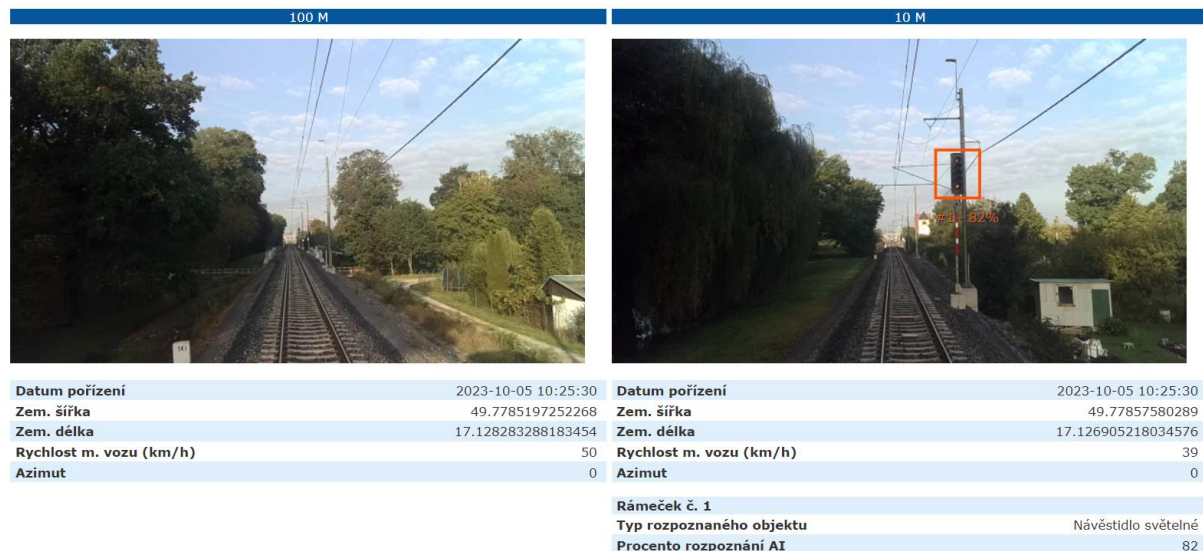
Obr. č. 7 - Detail návěstidla se snímky ze vzdálenosti 100 m a 10 m s AI detekcí
