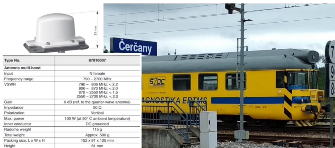
Obr. 1 - Motorový měřicí vůz ERTMS s použitými anténami
