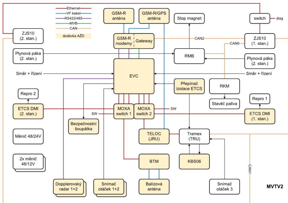
Obr. 1 – Příklad zapojení ETCS na vozidlech řady MVTV 2
